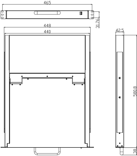
图 1-1.2 尺寸图
