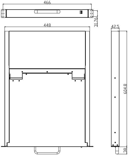
图 1-1.4 尺寸图
